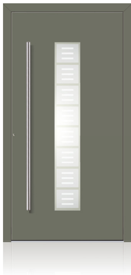
Enna | verglast in Ausführung Aufsatzfüllung Farbvariante Quarzgrau Sandstrahlung Enna 3 auf Grundglas Klarglas Teilflächen 1-fach sandgestrahlt Teilflächen 2-fach sandgestrahlt Teilflächen klar + Rand umlaufend 20 mm klar Artikel-Nr. E26 mit integriertem Griff HA 591 Edelstahl matt gebürstet
